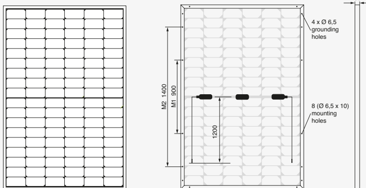
Abb. Prinzipskizze
